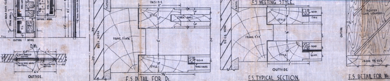
E.S. DETAIL FOR D1
