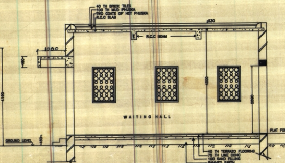
SECTION C-D
